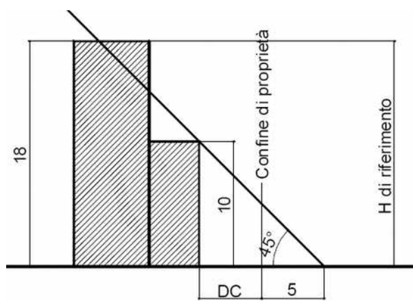
CASO 2 – Distanza dai confini = 18-5 = 13 mt
