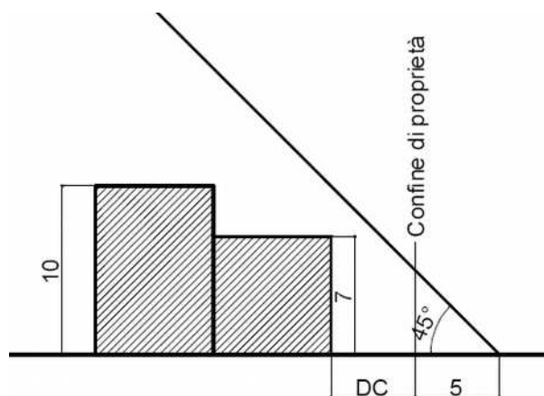
CASO 1 – Distanza dai confini = 5 mt
